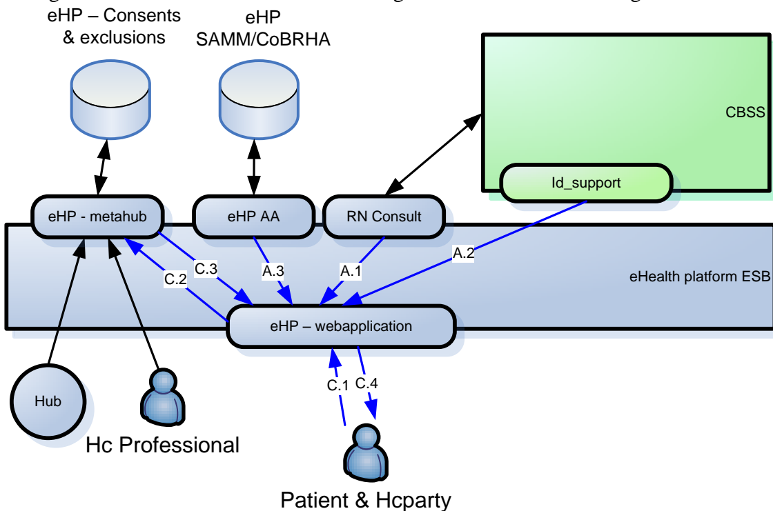
Figuur 1 : overzicht van de gegevensstromen voor het beheer van de toestemmingen
