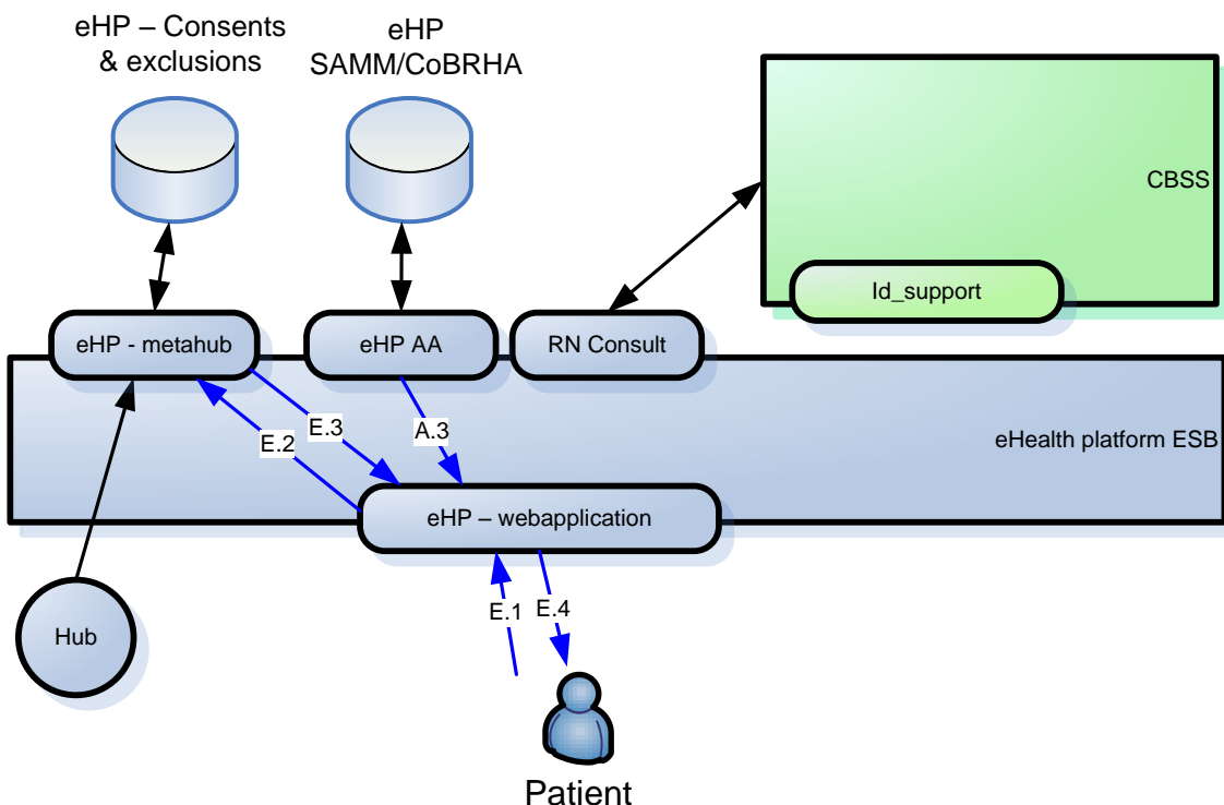
Figuur 2: overzicht van de gegevensstromen voor het beheer van de uitsluitingen
