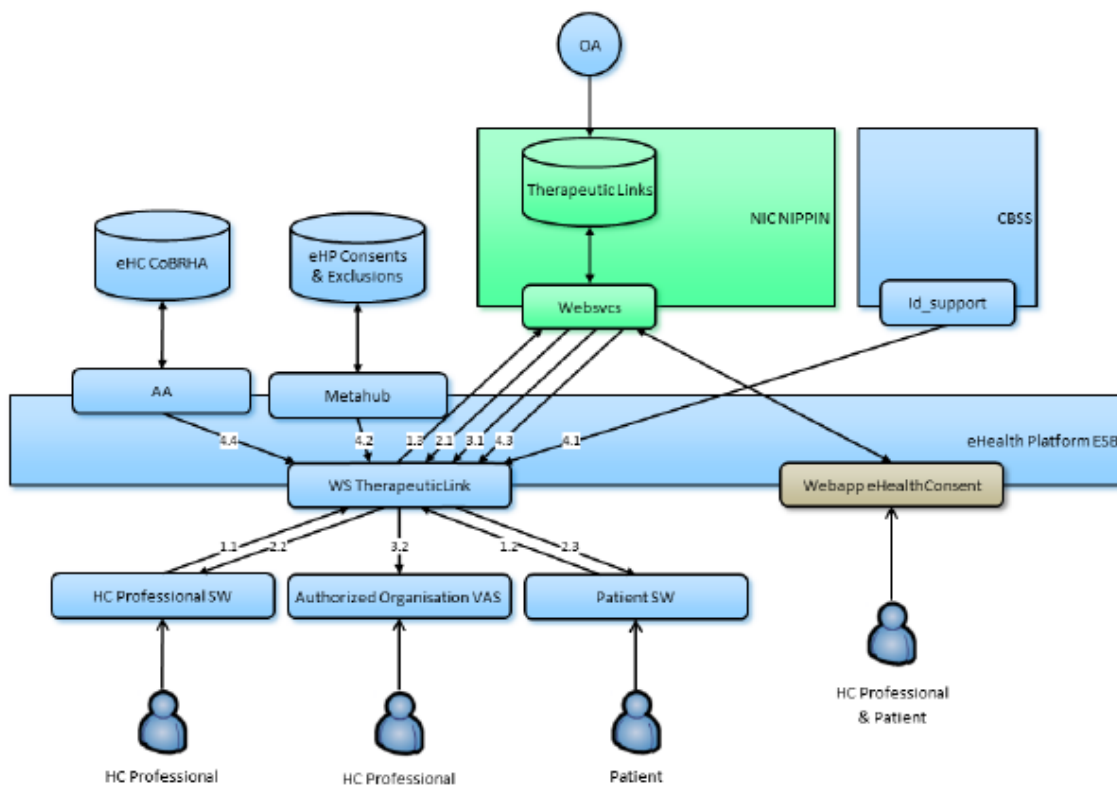
Figuur 4 : overzicht van de stromen in het kader van de webservice
